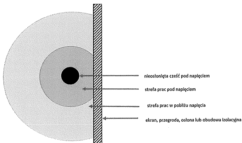
Rysunek Nr 2. Ograniczenie minimalnego odstępu w powietrzu poprzez zastosowanie sprzętu ochronnego
